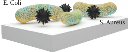
E. Coli
